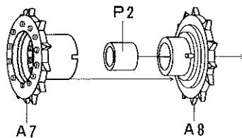
Drive Sprocket
