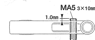
★MA5は図の位置で取り付けます。 ★Attach MA5 as shown. ★MA5 wie gezeigt anbauen. ★Fixer MA5 comme montré.
